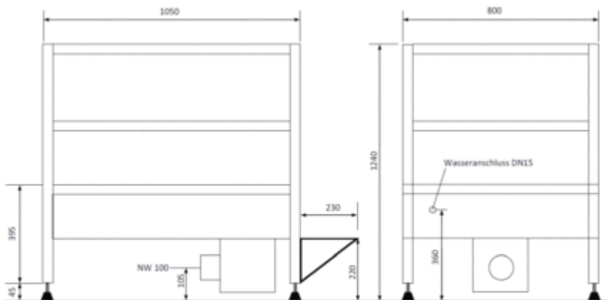
Stiefelwaschanlage STW 337-G Maßdetails
